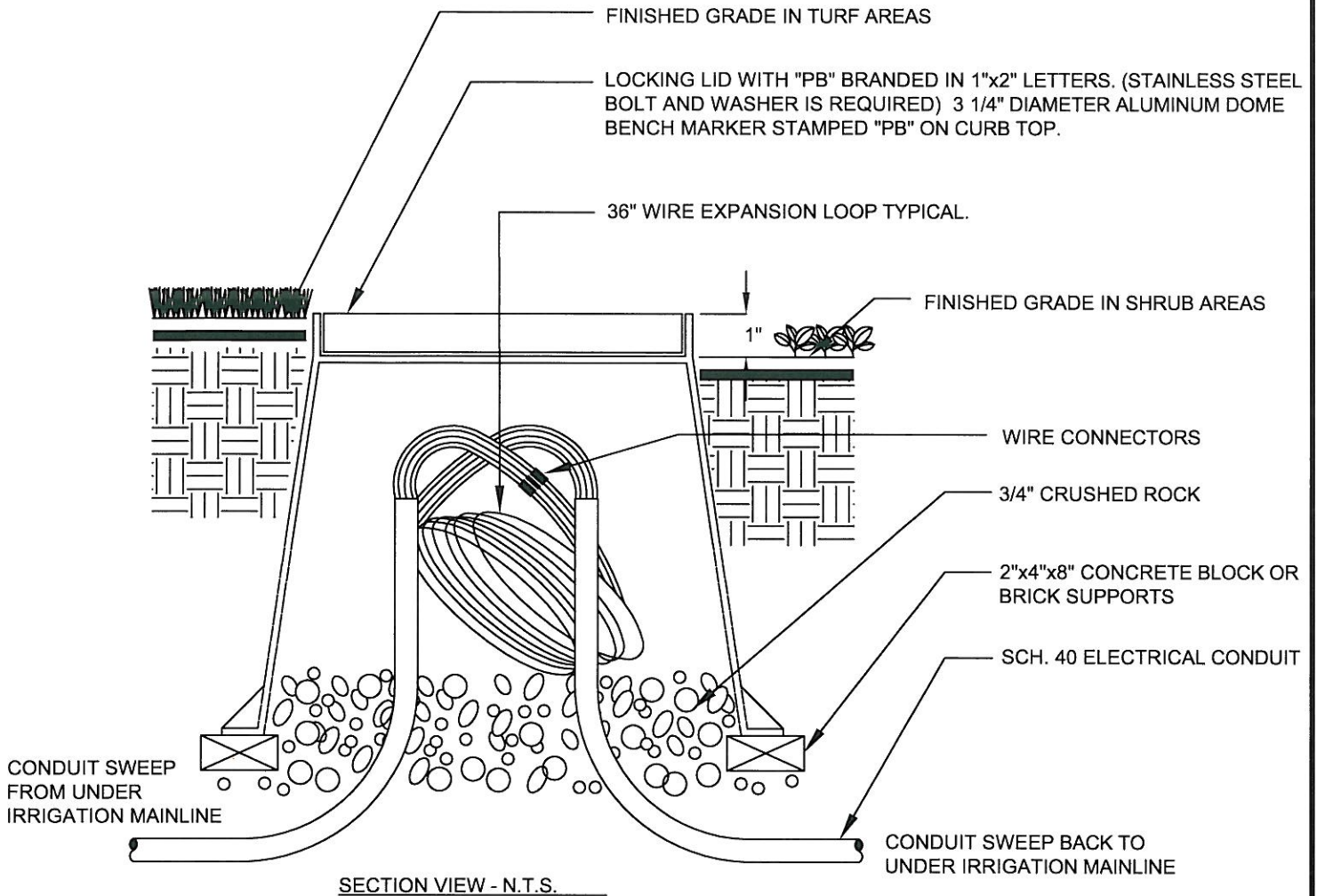
SECTION VIEW - N.T.S.
